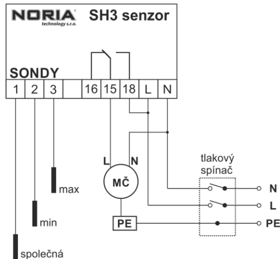
Příklad zapojení č.2: zapojení s tlakovým spínačem
