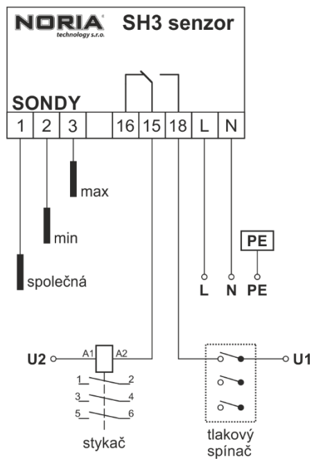
Příklad zapojení č.4: ovládání stykače tlakovým spínačem a beznapětovým kontaktem
