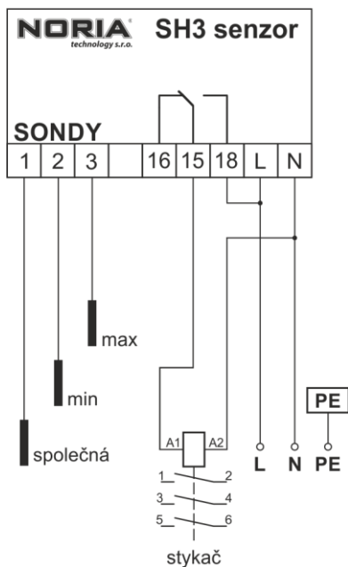
Příklad zapojení č.3: ovládání stykače
