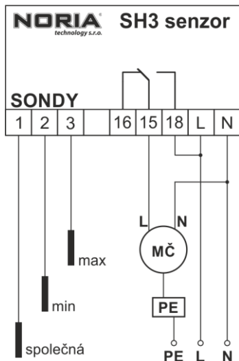
Příklad zapojení č.1: připojení jednofázového čerpadla
